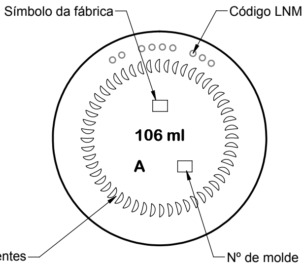
VISTA DO FUNDO / DE FONDO BOTTOM VIEW
